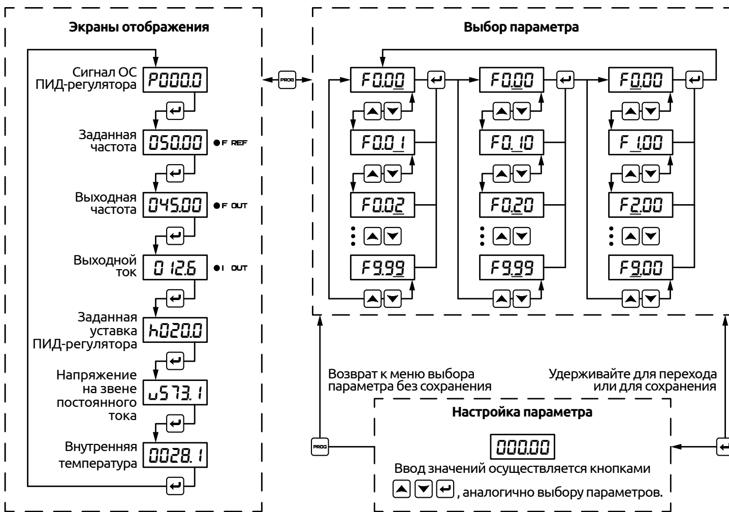
Рисунок 4 — Блок-схема навигации пульта управления
