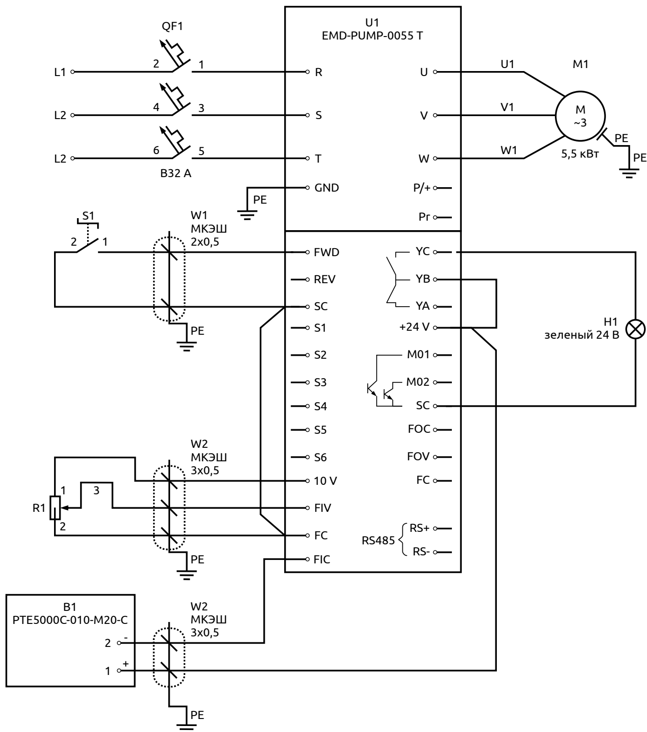
Рисунок 1 – Схема подключения ПЧ для управления насосом
